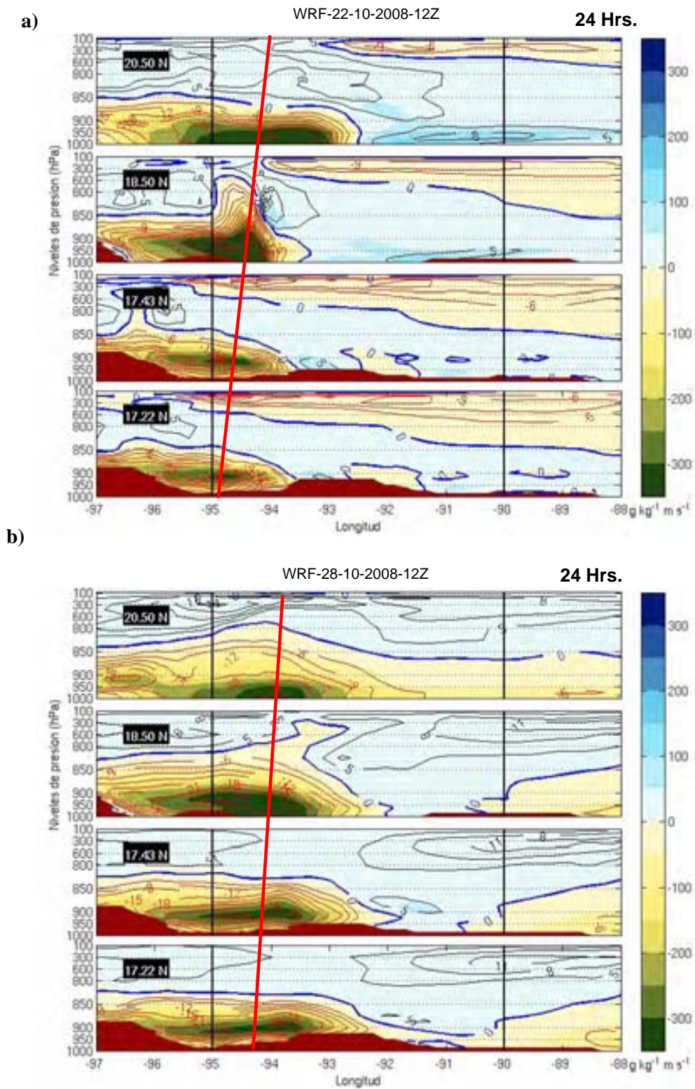
Figura 4.25. Cortes zonales para las latitudes mostradas en la figura 4.24. a) Pronóstico a 24 horas del día 22 de octubre. b) Pronóstico a 24 horas del día 28 de octubre. Áreas en color: Valores negativos (positivos) indican transporte de humedad hacia el sur (norte). Las líneas de contorno indican la intensidad de la componente meridional del viento: Rojo (negro) indica dirección hacia el sur (norte), la línea azul indica el cero. Las líneas negras verticales indican el rango de longitudes en las cuales se concentran las estaciones.
