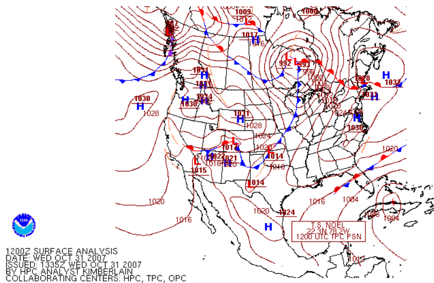
Figura 4.31. Análisis de superficie del día 28 de octubre a las 12Z.
