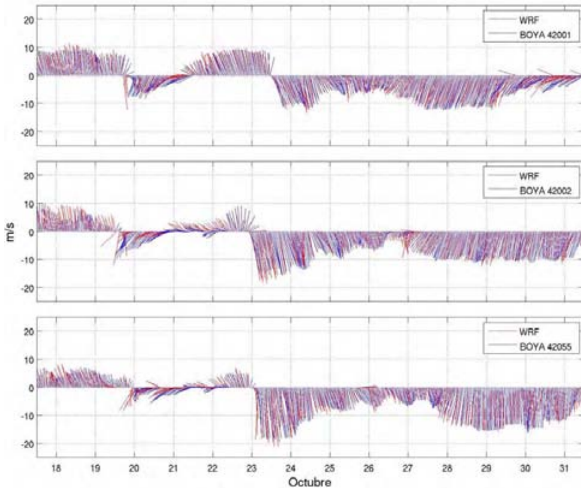
Figura 4.7. Comparación entre los vectores de viento a 10 m obtenidos con el modelo WRF en los puntos interpolados en las coordenadas de las boyas (rojo) y las observaciones en las boyas del NDBC ubicadas en el Golfo de México (azul), del 17 al 31 de octubre del 2007.
