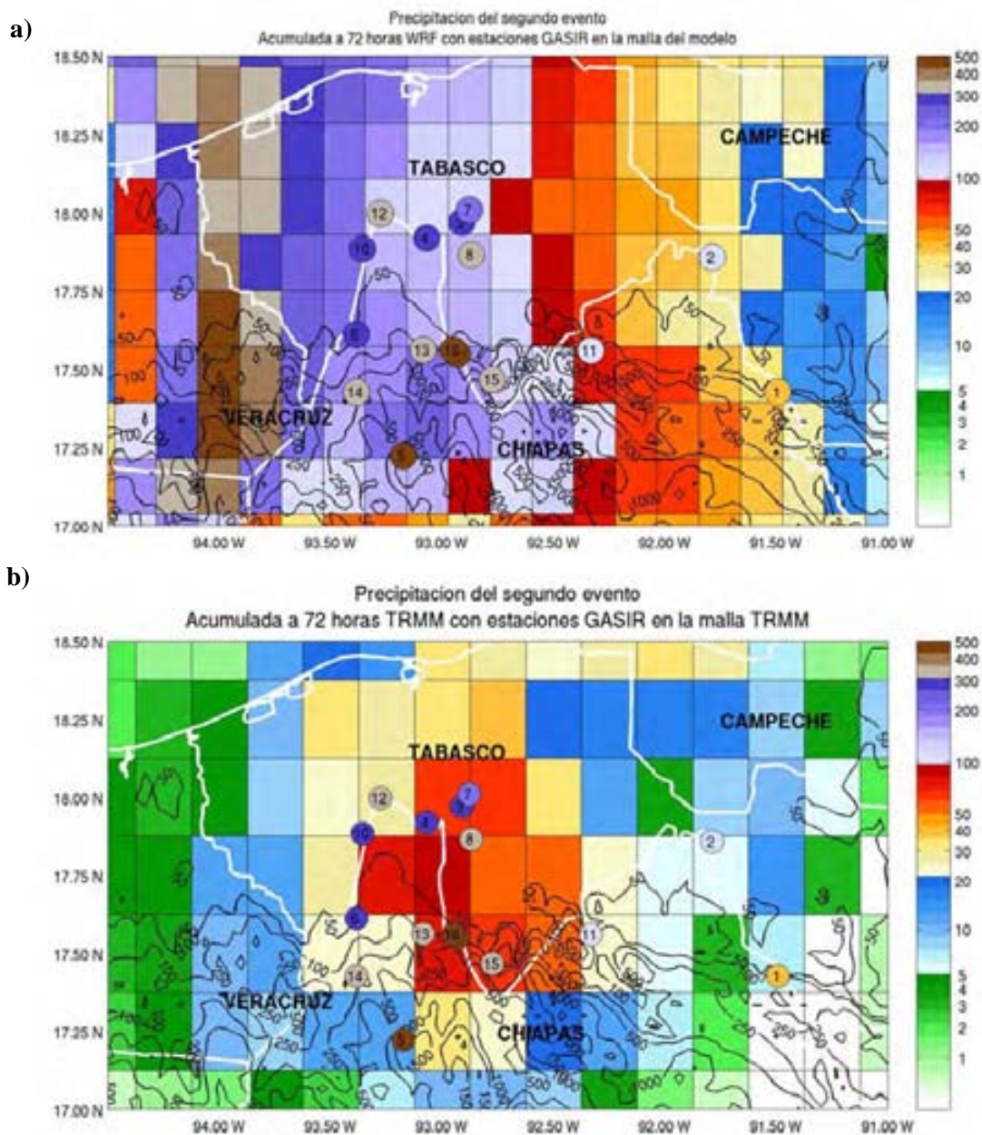
Figura 4.23. a) Precipitación acumulada en 72 horas estimada por el WRF a partir del 28-10-2007-12Z. b) Precipitación acumulada estimada por el TRMM del 22-10-2007-12Z al 25-10-2007-12Z. En ambos casos se muestran las observaciones registradas identificando las estaciones de acuerdo con la Tabla 2.2.
