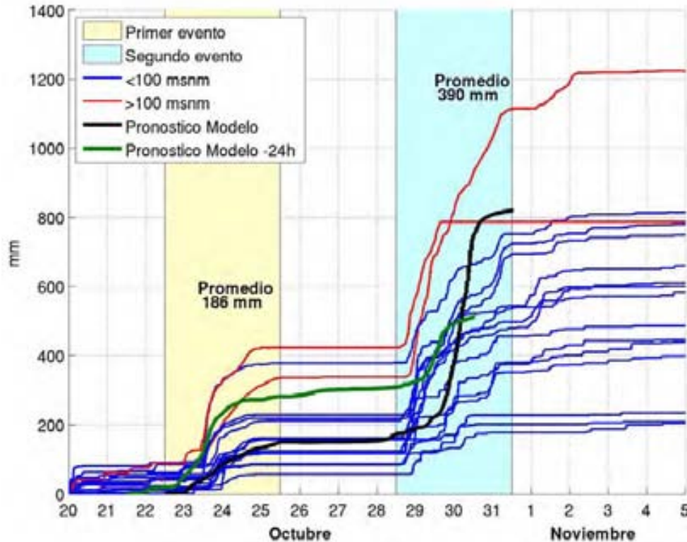
Figura 4.29. Precipitaciones acumuladas en las estaciones de la GASIR del 20 de octubre al 5 de noviembre. Las áreas sombreadas representan las 72 horas de precipitación de cada evento. La línea negra representa las precipitaciones acumuladas a 72 horas de los pronósticos del día 22, 25 y 28 de octubre. La línea es construida igual que la anterior, pero representa los pronósticos del día 21, 24 y 27 de octubre.
