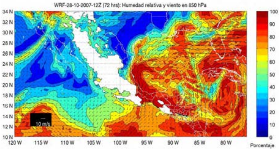
Figura 4.32. Humedad relativa y viento en 850 hPa. WRF-28-10-2007-12Z, pronóstico a 72 horas.
