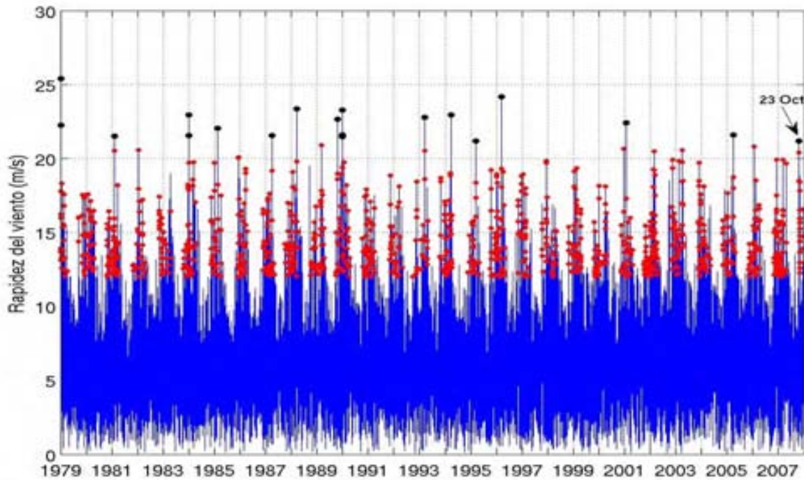
Figura 4.4. Rapidez del viento a 10 m cada 6 horas de los datos del NCEPR2 en el punto 20°N, 93.75°W para el periodo 1979-2007. Los puntos rojos indican la ocurrencia de eventos de norte , de acuerdo con la definición utilizada en este trabajo, y los puntos negros indican eventos con una intensidad similar a la del día 23 de octubre. Las líneas horizontales indican intensidades de viento entre 12 y 20 m/s.
