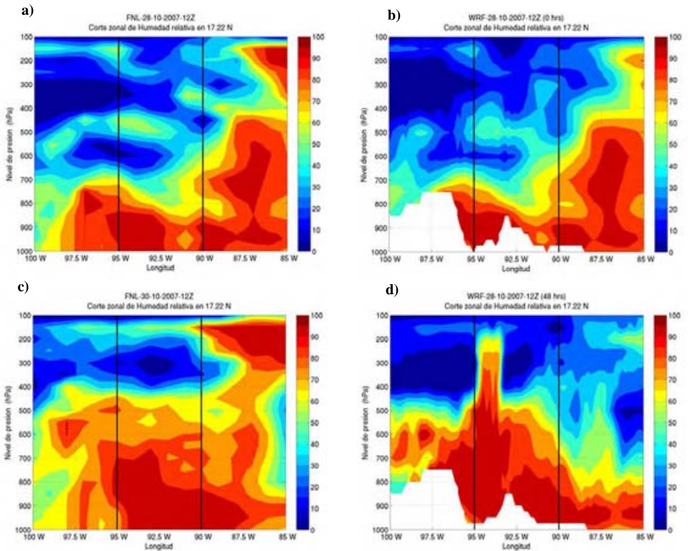
Figura 4.21. Cortes zonales de humedad relativa en 17.22 °N (latitud de Ocoatepec, Chiapas). a) FNL-28-10-2007-12Z. b) WRF 23-10-2007-12Z, condiciones iniciales. c) FNL-24-10-2007-00Z. d) WRF 23-10-2007-12Z, pronóstico a 48 horas. Las líneas negras indican el rango de longitud en que se localizan las estaciones de la GASIR.
