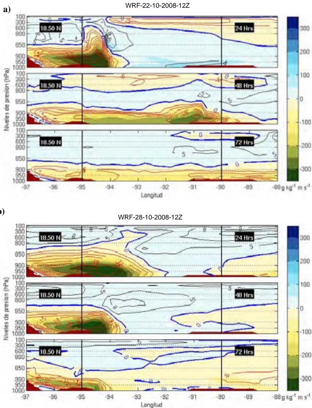
Figura 4.27. Cortes zonales como en 4.25. a) Pronóstico a 24, 48 y 72 horas del día 22 de octubre. b) Pronóstico a 24, 48 y 72 horas del día 28 de octubre.
