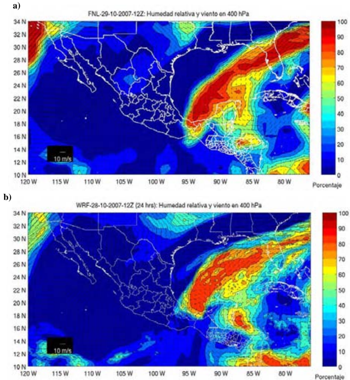
Figura 4.20. Humedad relativa y viento en 400 hPa. (a) FNL-29-10-2007-12Z. (b) WRF-28-10-2007-12Z, pronóstico a 24 horas.
