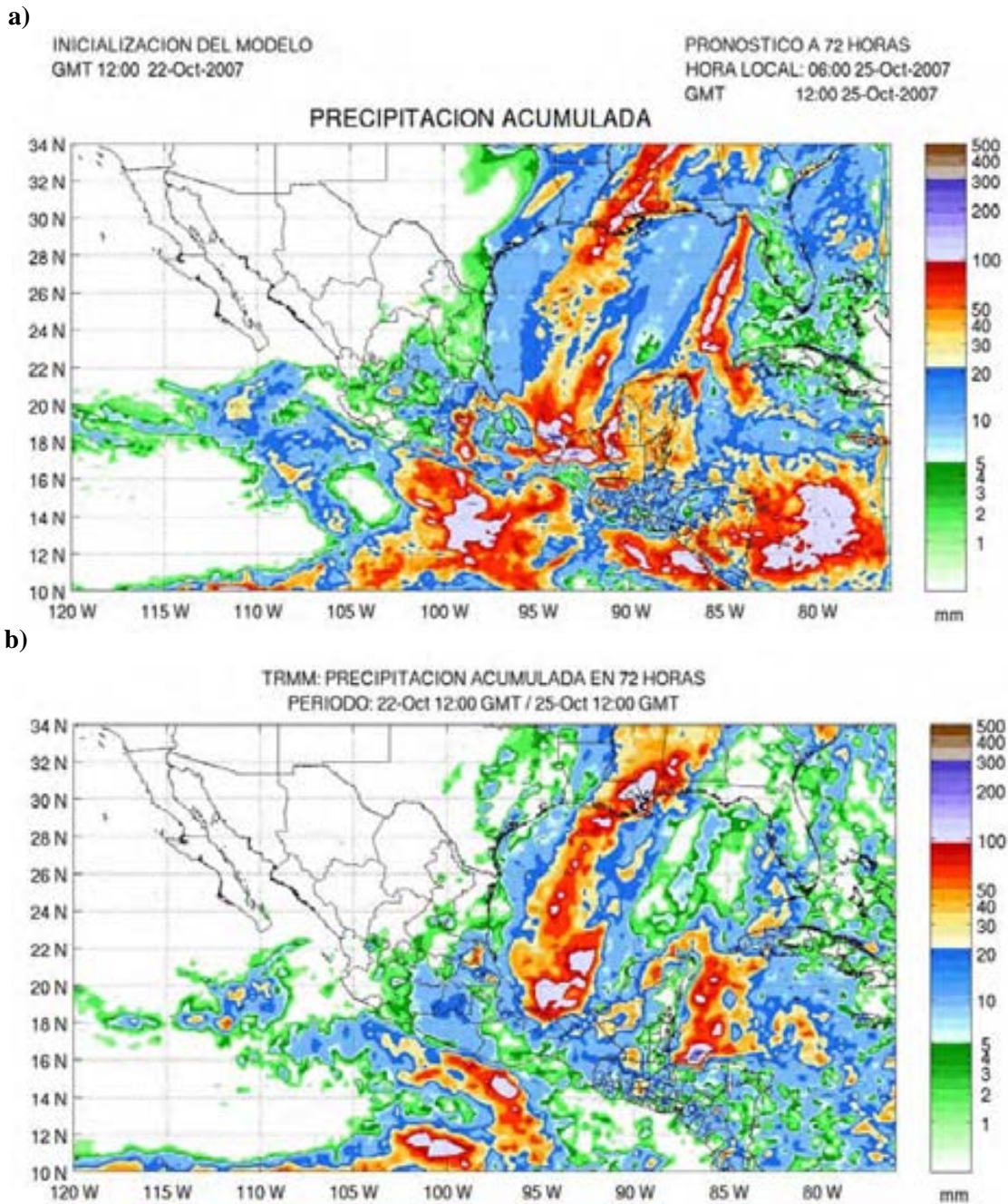
Figura 4.15. a) Precipitación acumulada en 72 horas estimada por el WRF a partir de 22-10-2007-12Z. b) Precipitación acumulada estimada por el TRMM del 22-10-2007-12Z al 25-10-2007-12Z.
