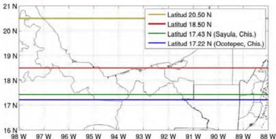
Figura 4.24. Latitudes utilizadas para realizar los cortes zonales.
