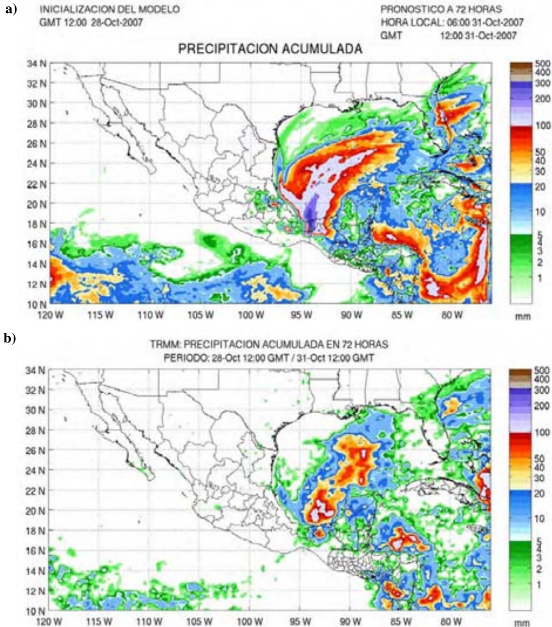
Figura 4.22. a) Precipitación acumulada en 72 horas estimada por el WRF a partir del 28-10-2007-12Z. b) Precipitación acumulada estimada por el TRMM del 28-10-2007-12Z al 31-10-2007-12Z.
