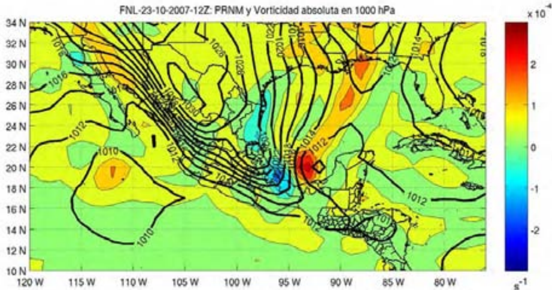
Figura 4.11. Presión reducida al nivel del mar (hPa) y vorticidad absoluta ( s^{-1} ) en 1000 hPa. FNL-23-10-2007-12Z.
