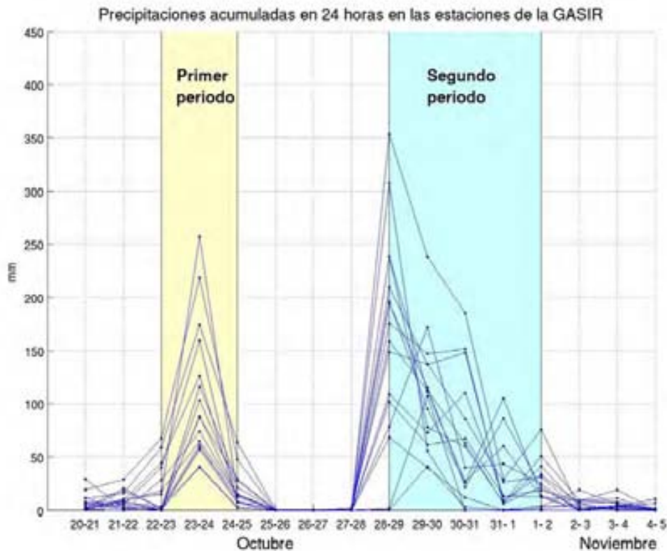
Figura 4.9. Precipitaciones diarias acumuladas en las estaciones de la GASIR del 20 de octubre al 5 de noviembre del 2007. Se observan dos periodos de precipitación intensa, el primero del 22 al 25 de octubre y el segundo del 28 de octubre al 2 de noviembre.
