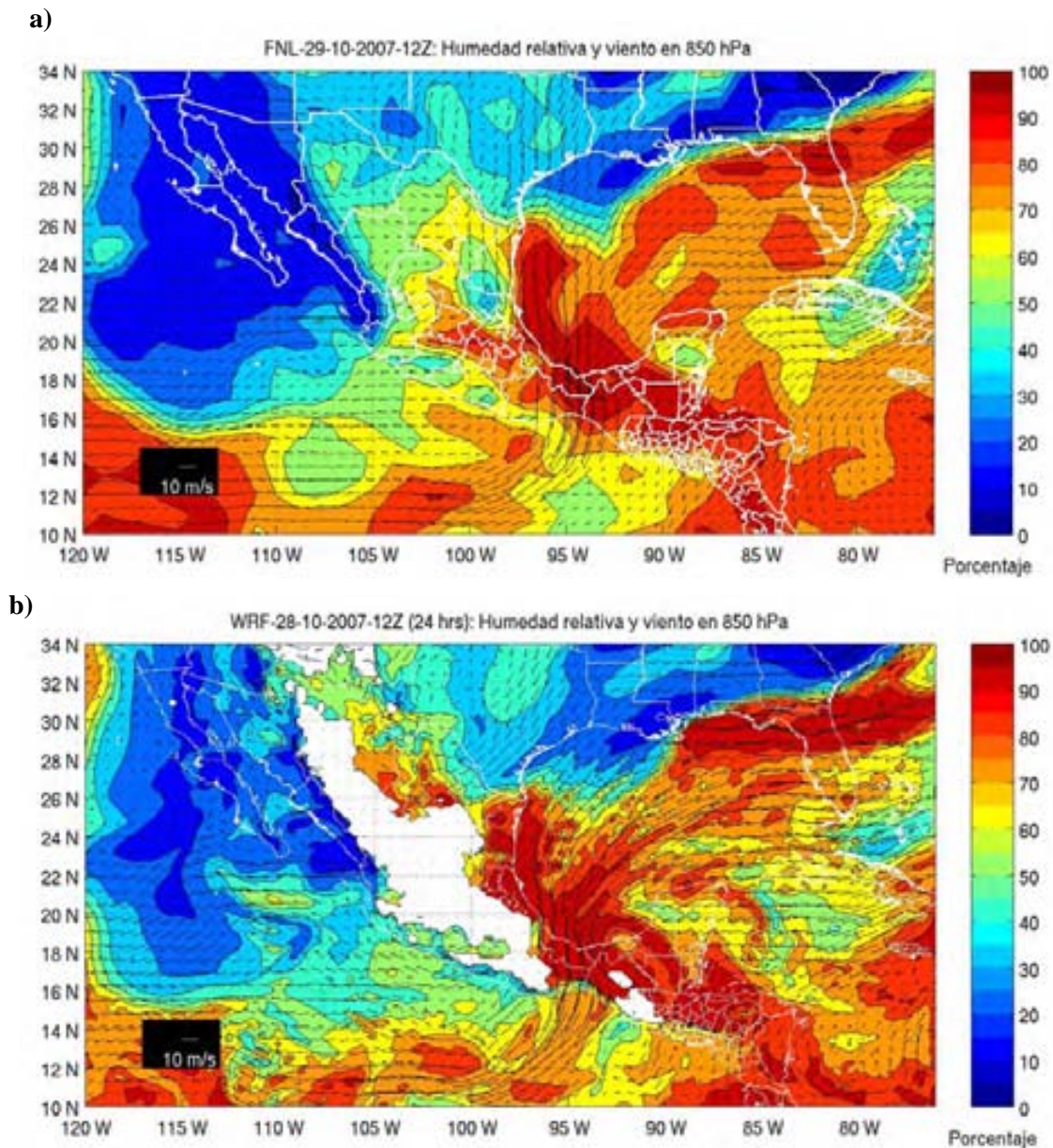
Figura 4.18. Humedad relativa y viento en 850 hPa. (a) FNL-29-10-2007-12Z. (b) WRF-28-10-2007-12Z, pronóstico a 24 horas.
