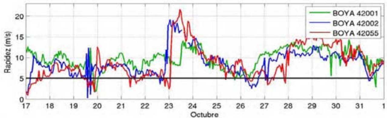
Figura 4.6. Observaciones horarias de la rapidez del viento a 10 m en las boyas del NDBC del 17 al 31 de octubre del 2007.
