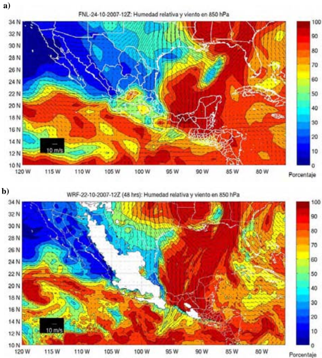
Figura 4.13. Humedad relativa y viento en 850 hPa. a) FNL-24-10-2007-12Z. b) WRF: 22-10-2007-12Z, pronóstico a 48 horas.
