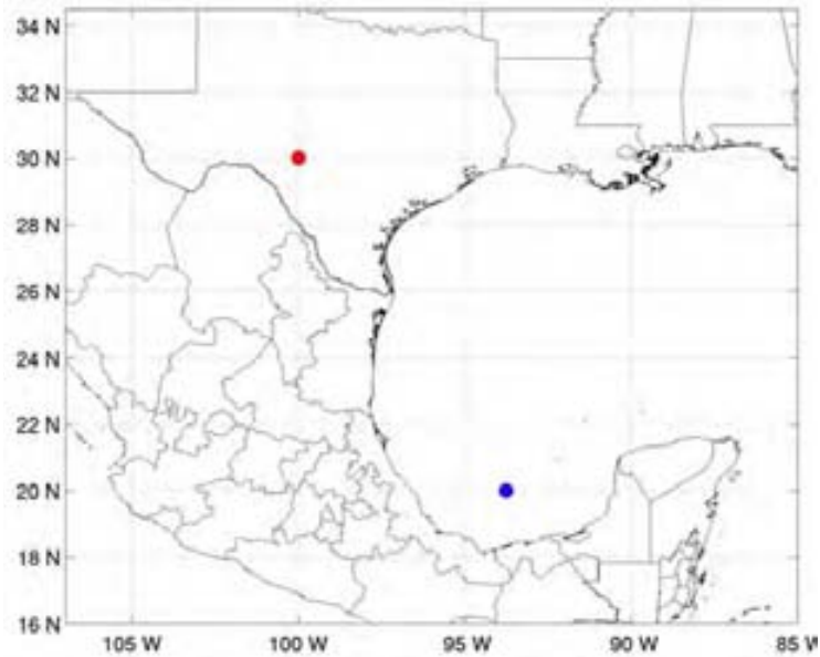
Figura 4.3. Puntos tomados como referencia para definir un norte (ver texto principal).
