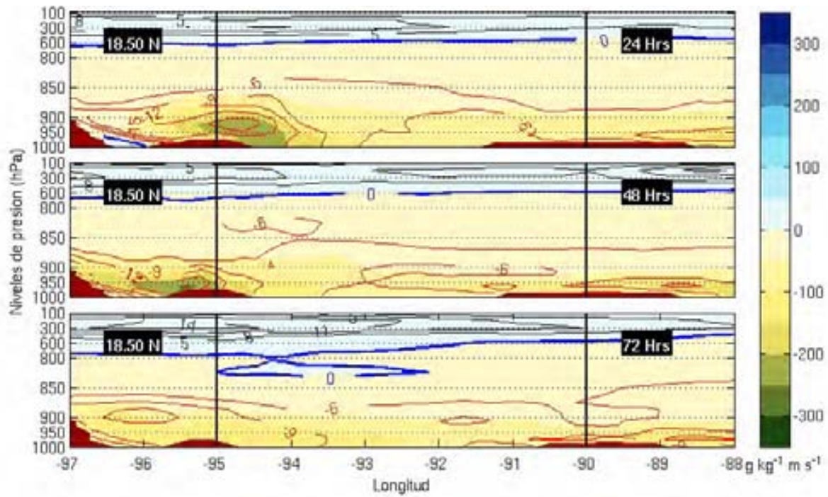
Figura 4.35. Cortes zonales como en 4.25. Pronóstico a 24, 48 y 72 horas del día 31 de octubre.
