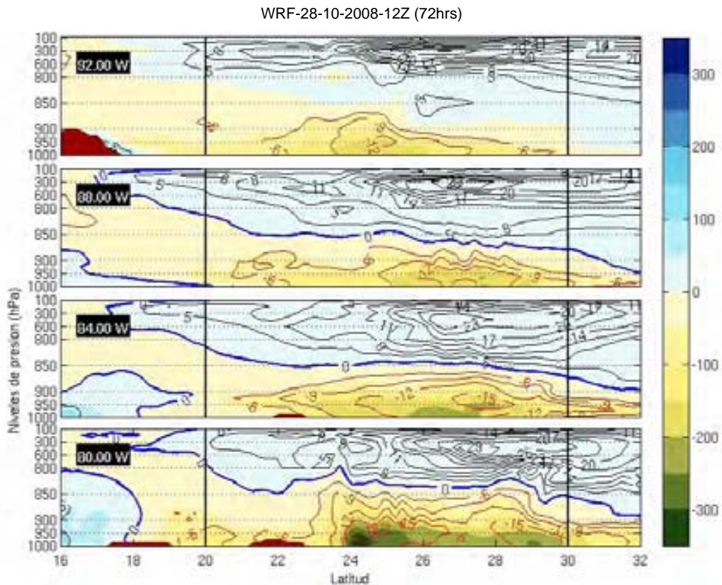
Figura 4.33. Cortes meridionales para las longitudes mostradas en la figura 4.32. Pronóstico a 72 horas del 28 de octubre. Áreas en color: Valores negativos (positivos) indican transporte de humedad hacia el oeste (este). Las líneas de contorno indican la intensidad de la componente zonal del viento: Rojo (negro) indica dirección hacia el oeste (este), la línea azul indica el cero. Las líneas negras verticales indican el rango de latitud en el cual se ubica la tormenta tropical.
