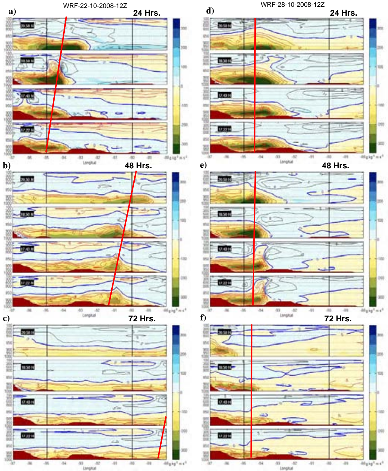
Figura 4.26. Cortes zonales igual que en 4.25. En (a), (b) y (c) se muestra el pronóstico a 24, 48 y 72 horas respectivamente, iniciando el modelo el día 22 de octubre. En (d), (e) y (f) se muestra el pronóstico a 24, 48 y 72 respectivamente, iniciando el modelo el día 28 de octubre.
