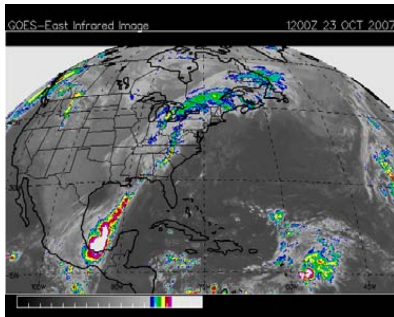
Figura 4.12. Imagen satelital infrarroja del 23-10-2007-12Z. Se observa un área de fuerte convección sobre la Bahía de Campeche debido a la interacción entre el sistema de alta presión y el pequeño sistema de baja presión en la zona.
