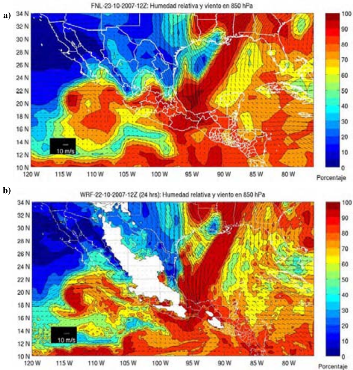
Figura 4.10. Humedad relativa y viento en 850 hPa. (a) FNL-23-10-2007-12Z. (b) WRF-22-10-2007-12Z, pronóstico a 24 horas.
