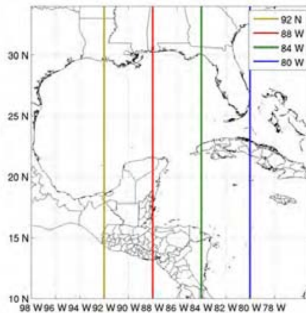
Figura 4.34. Longitudes utilizadas para realizar los cortes meridionales.
