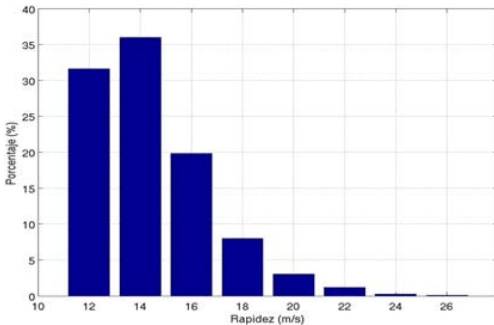
Figura 4.5. Distribución de frecuencias, como porcentaje de ocurrencia, de la rapidez del viento en los eventos de norte para el periodo 1979-2007 a partir de los datos del NCEPR2.
