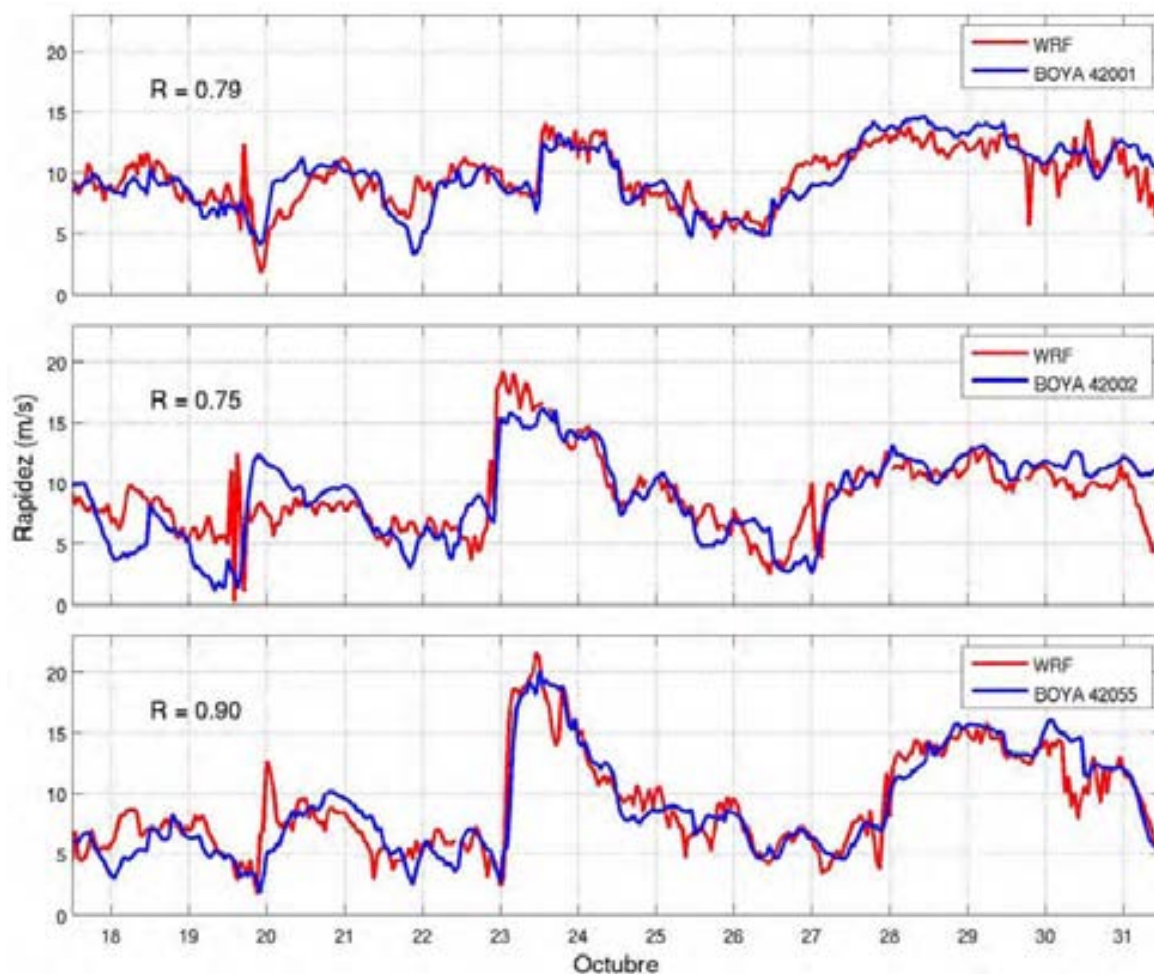
Figura 4.8. Correlación lineal entre los datos horarios de la rapidez del viento observado a 10 m en las boyas del NDBC y los obtenidos con el modelo del 17 al 31 de octubre. Los datos de las boyas se ilustran en color azul y en rojo los del modelo.
