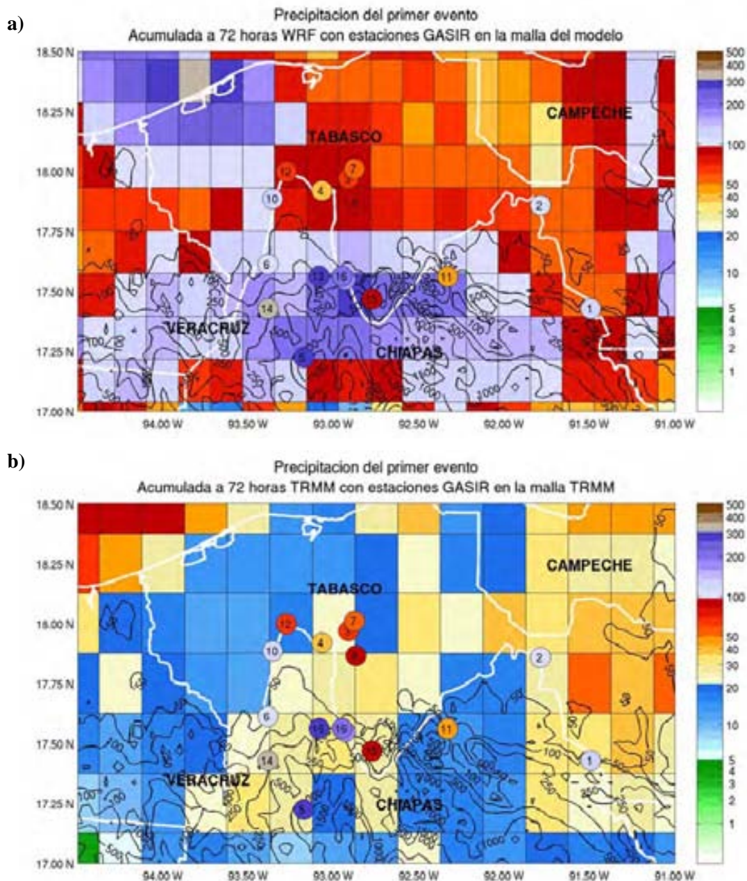
Figura 4.16. a) Precipitación acumulada en 72 horas estimada por el WRF a partir del 22-10-2007-12Z. b) Precipitación acumulada estimada por el TRMM del 22-10-2007-12Z al 25-10-2007-12Z. En ambos casos se muestran las observaciones registradas identificando las estaciones de acuerdo con la Tabla 2.2.
