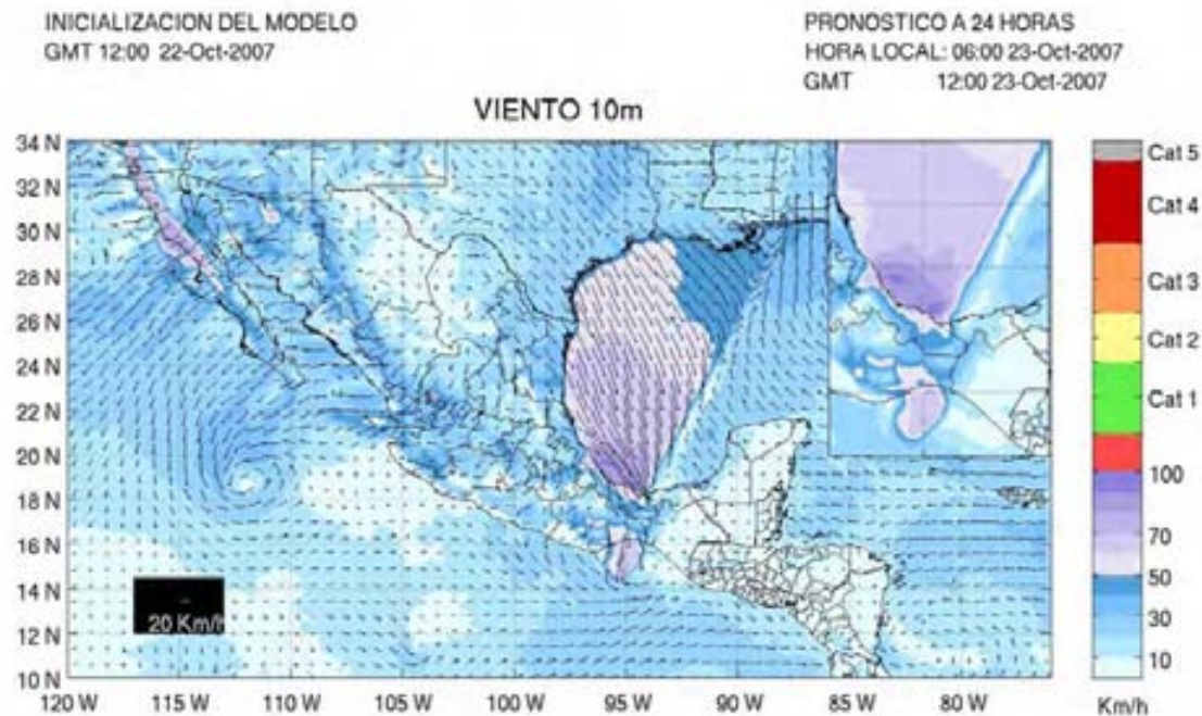
Figura 4.2. Pronóstico a 24 horas de la rapidez y dirección del viento a 10 m con el modelo WRF (WRF-22-10-2007-12Z).
