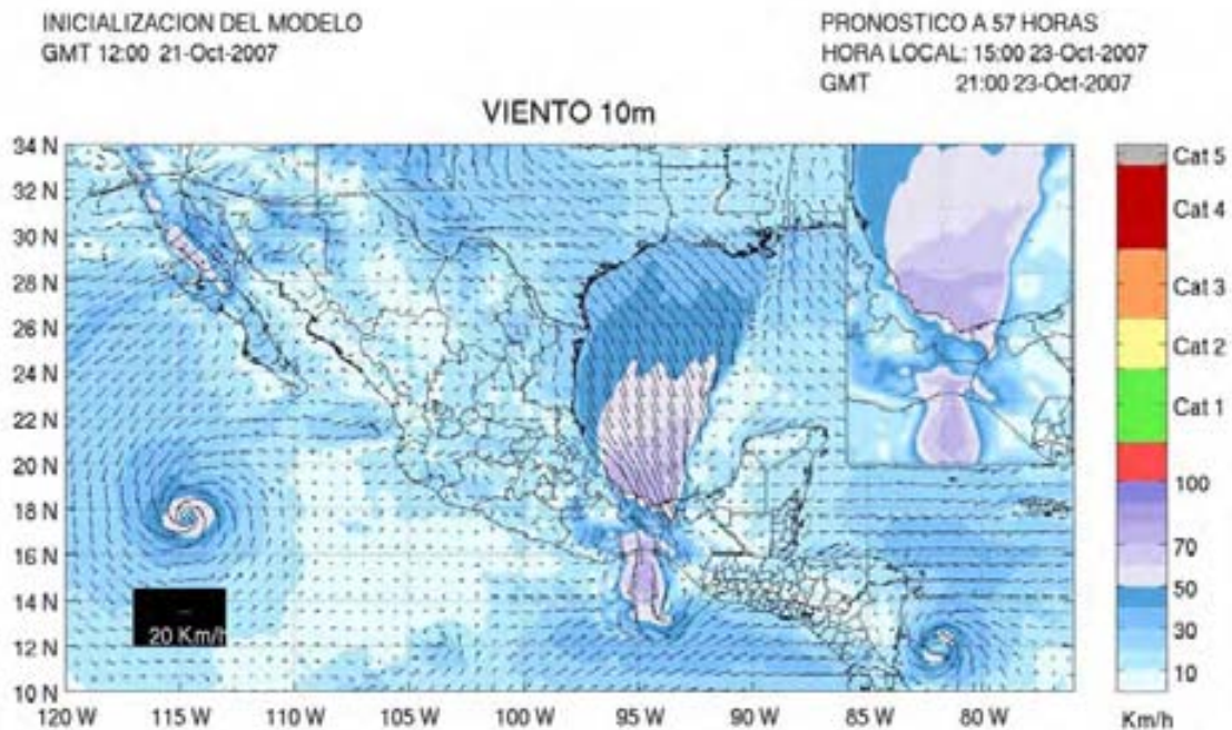
Figura 4.1. Pronóstico a 57 horas de la rapidez y dirección del viento a 10 m con el modelo WRF (WRF-21-10-2007-12Z).
