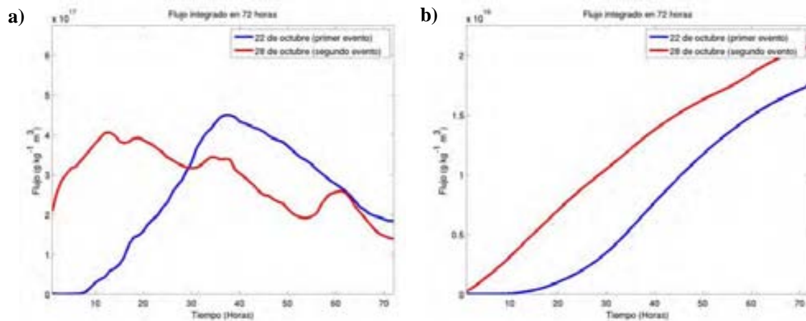
Figura 4.28. Flujo de vapor de agua para los dos eventos de precipitación durante 72 horas de pronóstico. a) Flujo horario. b) Flujo acumulado.
