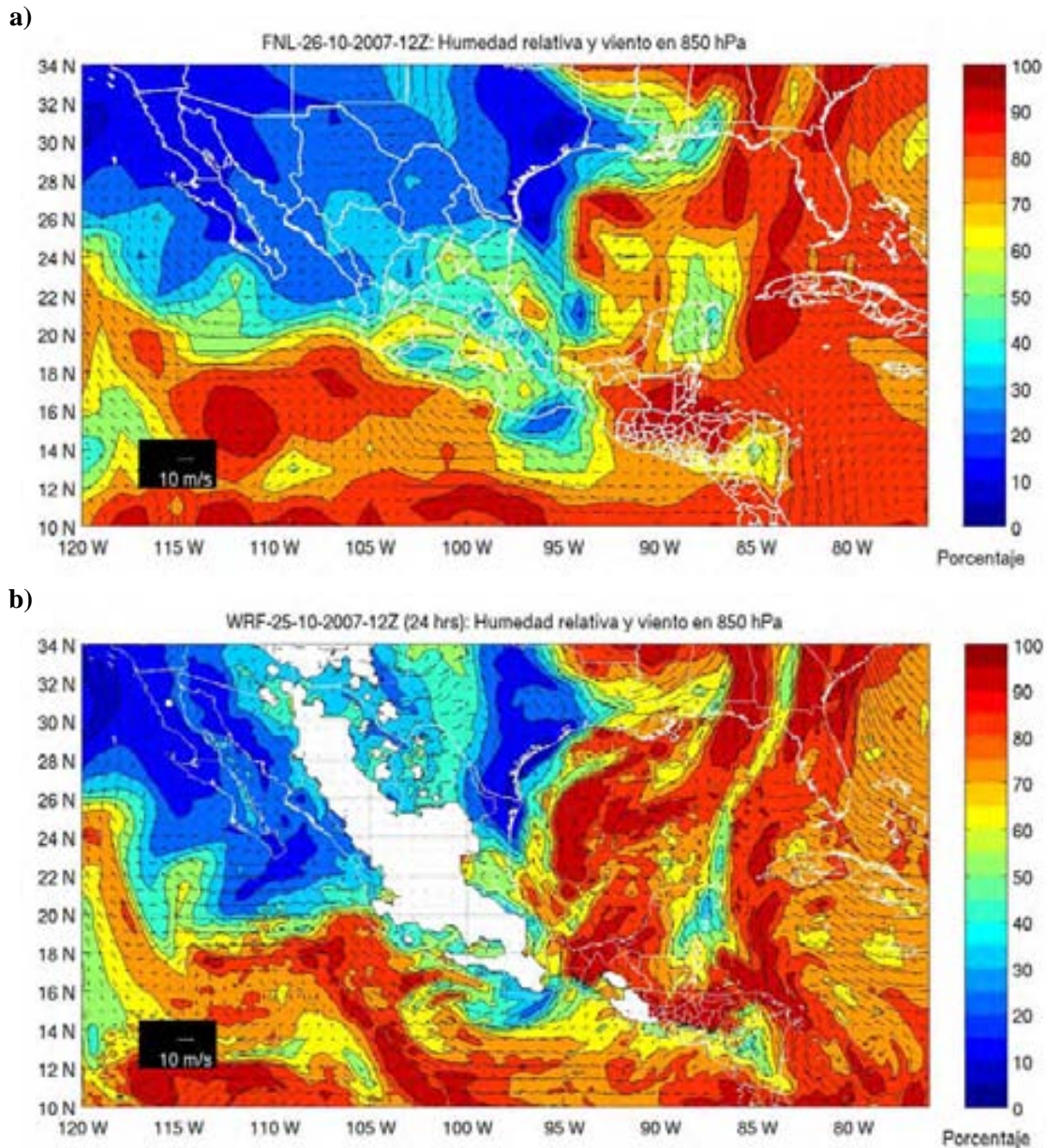
Figura 4.17. Humedad relativa y viento en 850 hPa. (a) FNL-26-10-2007-12Z. (b) WRF-25-10-2007-12Z, pronóstico a 24 horas.
