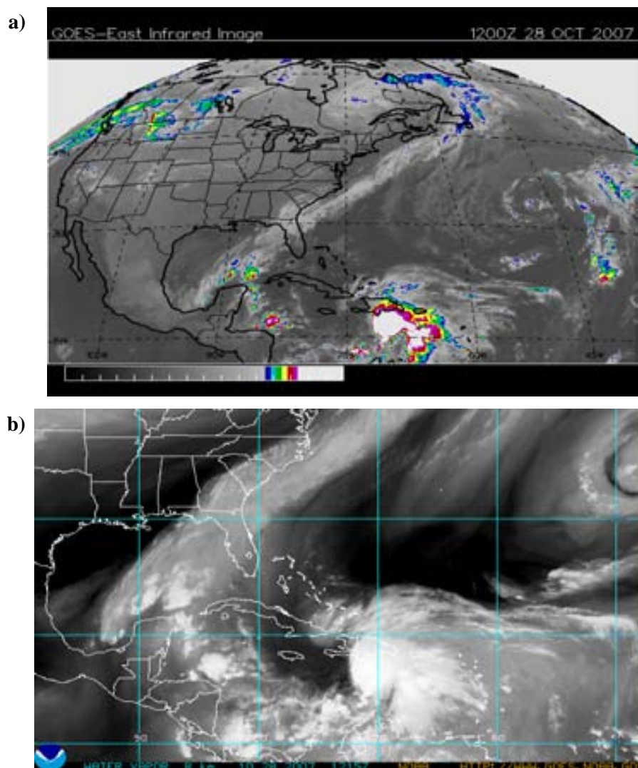
Figura 4.30. Imágenes satelitales del día 28 de octubre a las 12Z. a) Imagen infrarroja indicando la temperatura del tope de las nubes de acuerdo con la escala de la figura 1.2. b) Imagen de vapor de agua.
